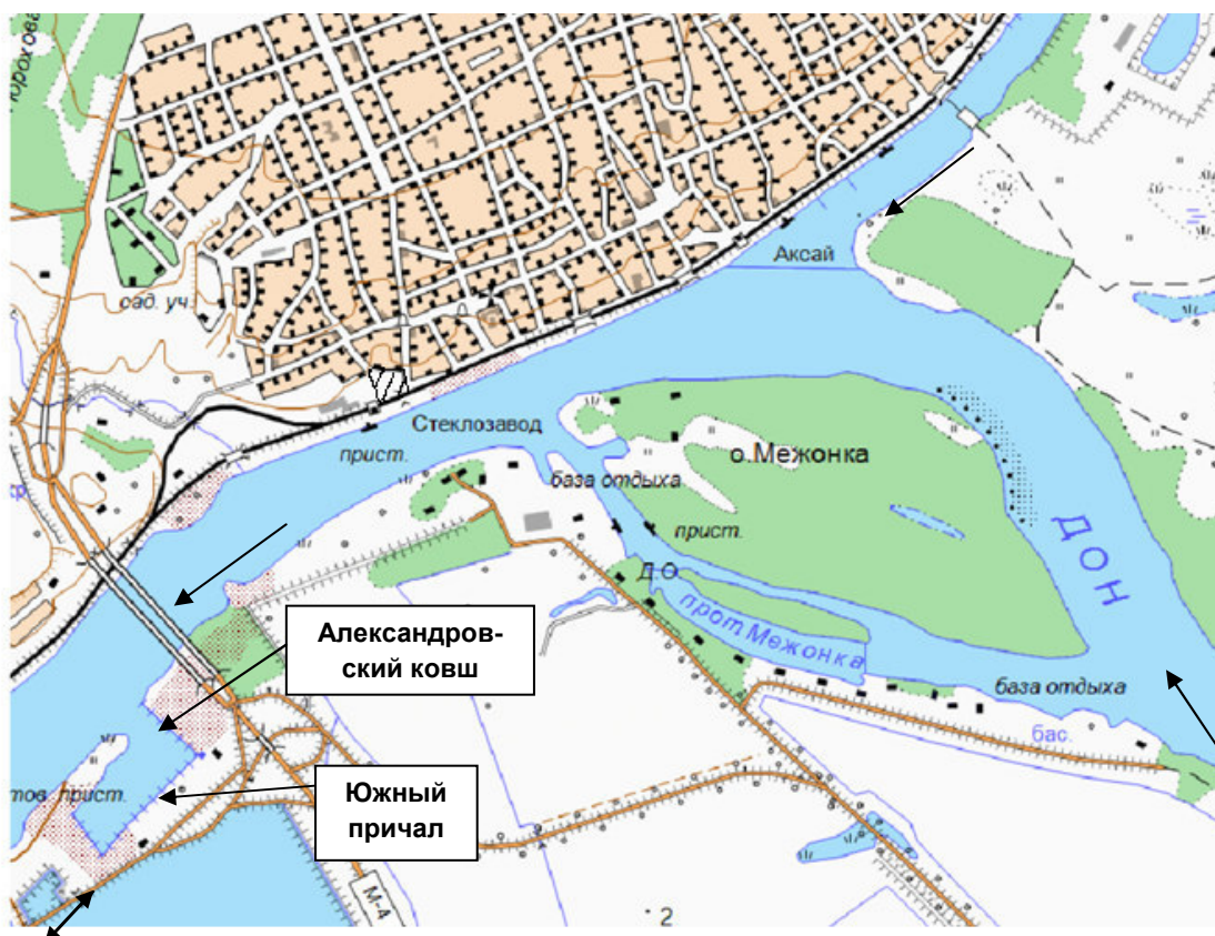
Рисунок 1 – Ситуационный план Южного причала
